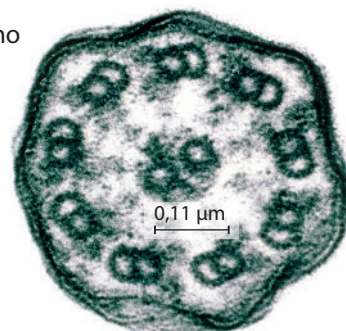
Figura 4.17. Eletromicrografia de um cílio cortado transversalmente. (Microscópio eletrônico de transmissão; aumento \approx 90.000\times .)
