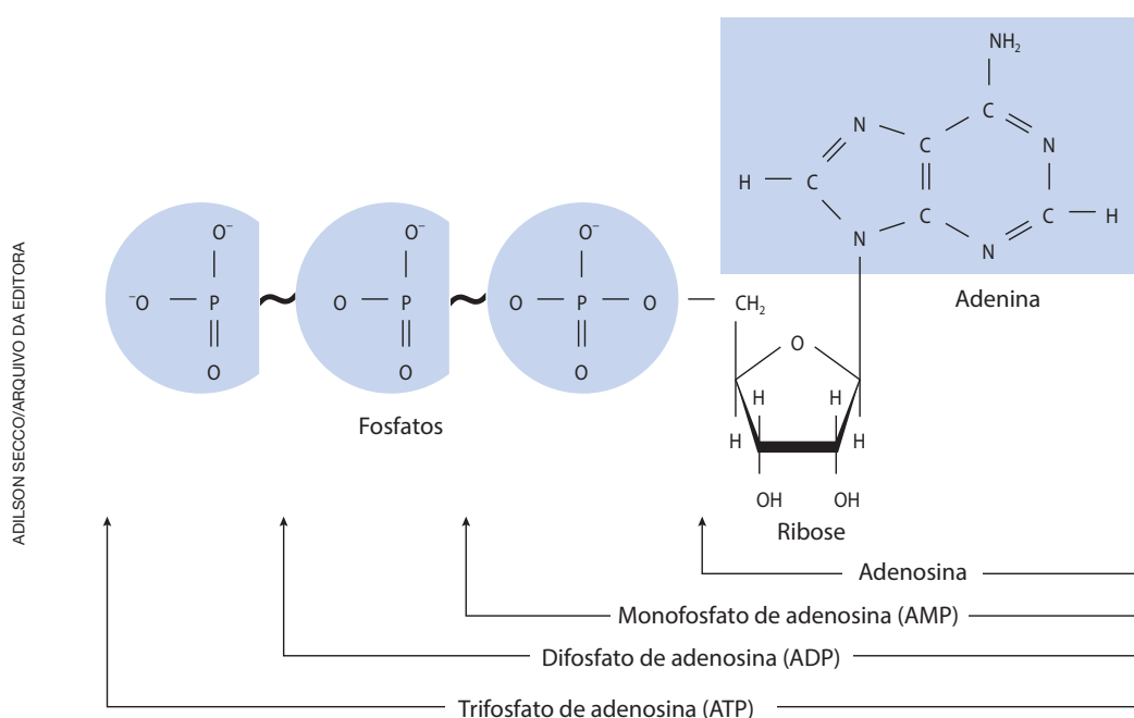
Figura 6.1. Fórmula estrutural do ATP. A parte da molécula do ATP formada pela adenina e pela ribose é chamada adenosina.
