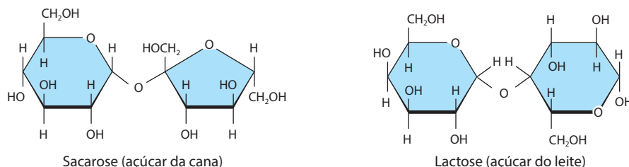
Figura 3.5. Fórmulas dos dissacarídios sacarose e lactose.
