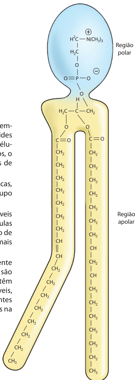
Figura 3.9. Estrutura molecular da fosfatidilcolina (lecitina), fosfolipídio componente das membranas das células vivas. A molécula de fosfolipídio apresenta uma extremidade polar unida a duas cadeias carbônicas apolares. (Representação fora de proporção; cores meramente ilustrativas).
