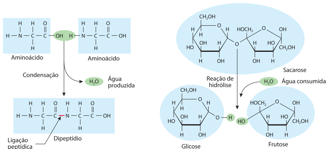
Figura 3.2. À esquerda, reação de condensação entre dois aminoácidos, uma síntese por desidratação. À direita, uma reação de hidrólise, em que a água participa como reagente na quebra molecular. No caso, a reação é a digestão do açúcar sacarose, que resulta em glicose e frutose.
