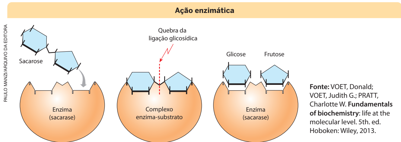
Figura 3.13. Representação esquemática de ação enzimática. A enzima sacarase liga-se a uma molécula de sacarose, promovendo a ruptura da ligação entre seus dois componentes: a glicose e a frutose. (Representação fora de proporção; meramente ilustrativas.)
