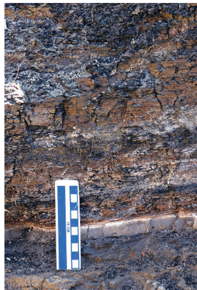
Figura 21.4. Corte de uma rocha sedimentar em Wyoming (EUA) em que há uma camada de sedimentos com alta concentração de irídio. Supõe-se que o irídio foi proveniente de um grande corpo celeste que teria se chocado com a Terra há 66 milhões de anos, causando a onda de extinções do final do período Cretáceo.
