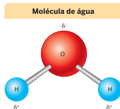
Figura 3.1. A molécula de água é polarizada. A região da molécula em que se localiza o átomo de oxigênio tem carga elétrica parcialmente negativa, representada por \delta^- , e a região em que se localizam os átomos de hidrogênio tem carga elétrica parcialmente positiva, simbolizada por \delta^+ . (Representação fora de proporção; cores meramente ilustrativas.)
